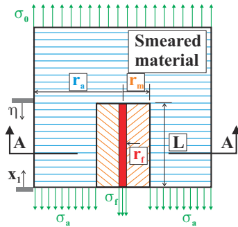
Fig. 2.13. Stress diffusion problem.
