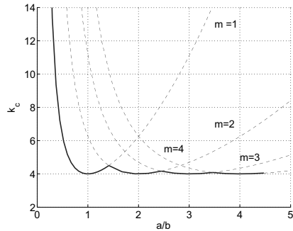
Fig. 16.51. Buckling parameter versus plate's aspect ratio.
