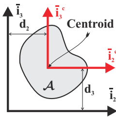
Fig. 6.9. Parallel axes.
