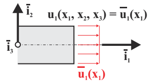
Fig. 5.7. Axial displacement distribution.
