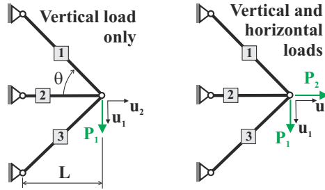
Fig. 10.16. Simple 3-bar truss.
