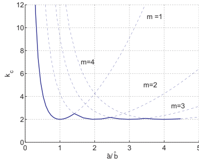
Fig. 16.52. Buckling parameter versus plate’s affine aspect ratio.
